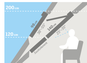
Klapp-Schwing-Fenster mit Untenbedienung
