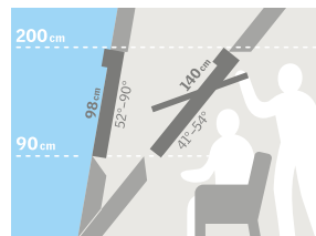
Schwingfenster mit Obenbedienung
